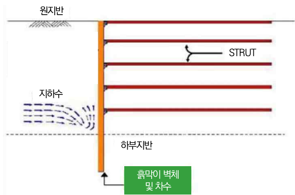
(a) 흙막이 벽체 및 차수적용
