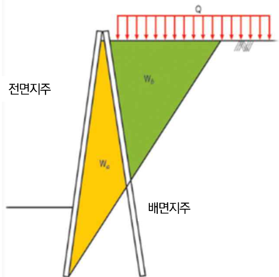
지주식 흙막이 토압 개념도
