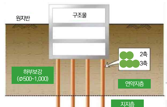
(d) 구조물 하부 보강공사
